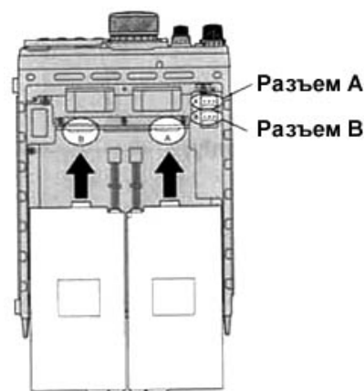
Разъем А Разъем В рисунок 3
