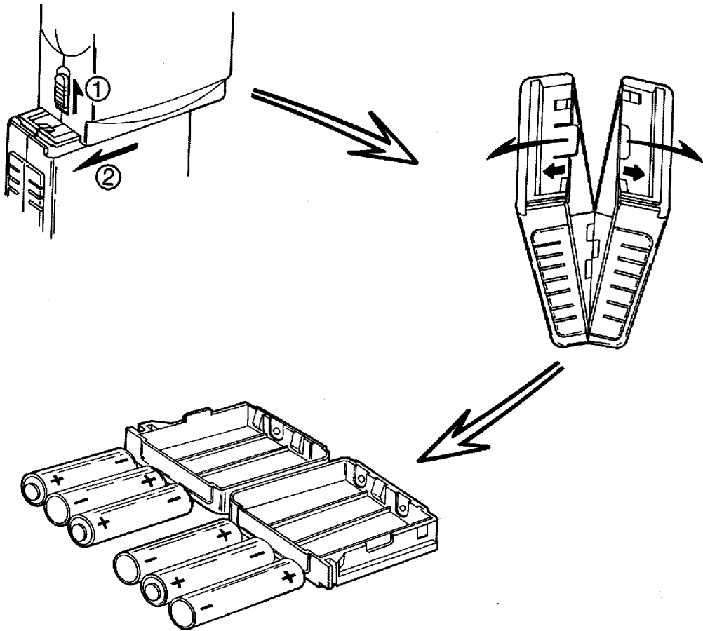
Рис 2. Батареи и батарейный отсек.
