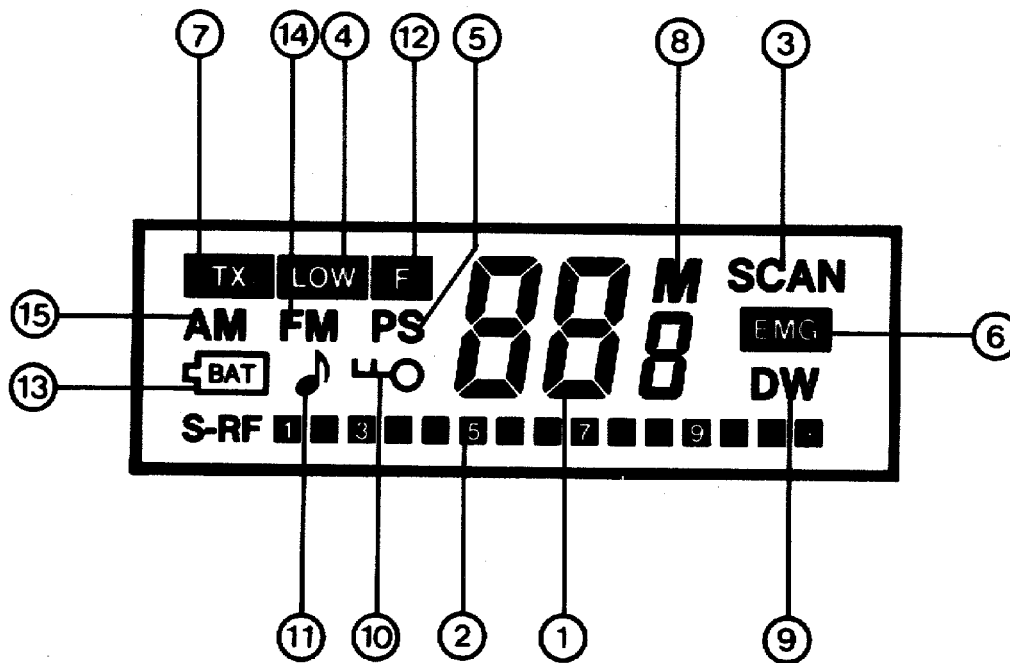
Рис. 5. Изображения мнемонических знаков ЖКИ-дисплея.
