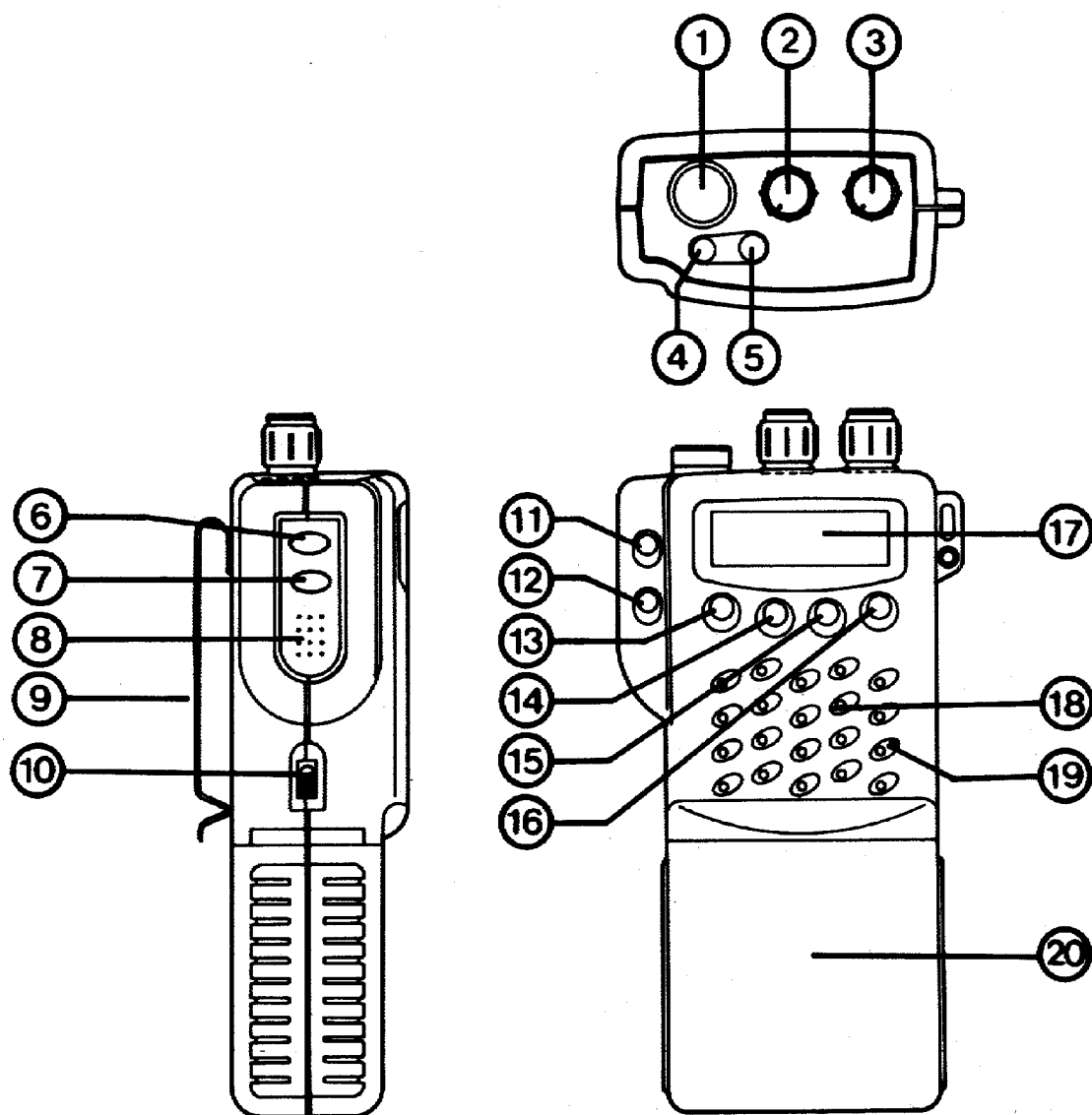
Рис. 1. Радиостанция Маусом АН-27 . Внешний вид.
