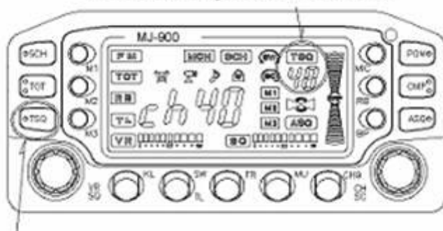
Кнопка тонового шумоподавителя TSQ (CTCSS)
