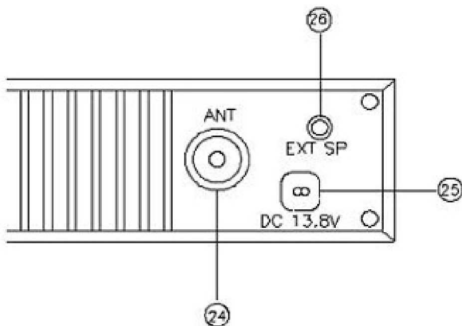
Задняя панель
