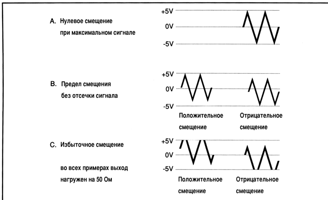
Рис. 4. Использование регулировки смещения по постоянному напряжению
