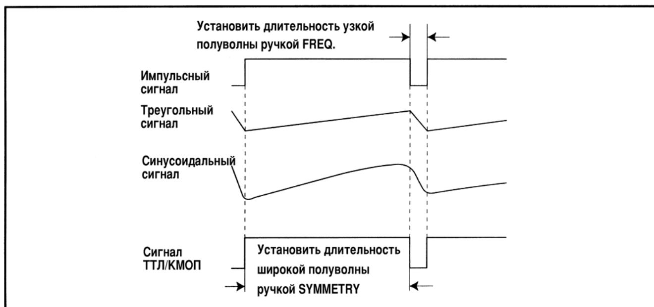
Рис. 5. Генерация прямоугольных, треугольных и синусоидальных сигналов
