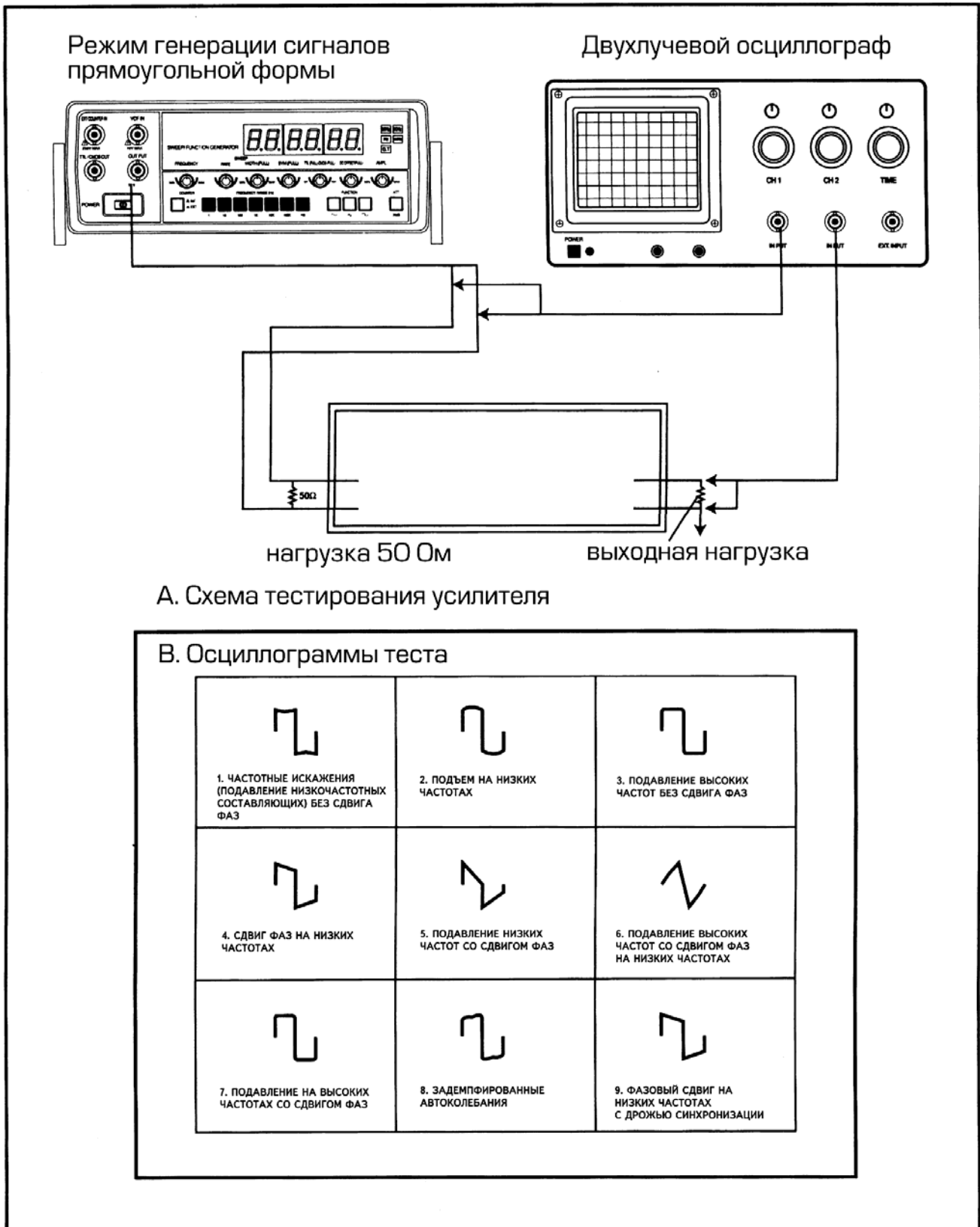
Рис 7. Оценка качества работы усилителя с помощью прямоугольных сигналов
