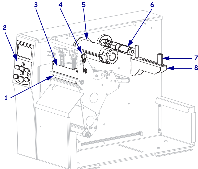
Рис. 1 • Компоненты принтера
