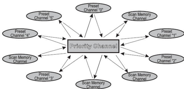
Сканирование Памяти
