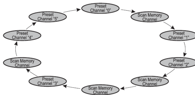
Приоритетное Сканирование
