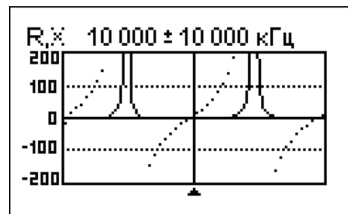
Короткозамкнутый кабель
