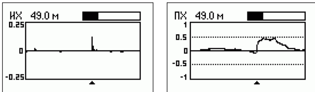
Графики импульсной и переходной характеристик
