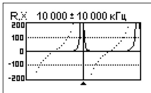
Разомкнутый кабель
