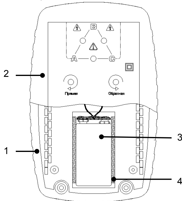
Рисунок 4.2 – Расположение батареи в указателе
