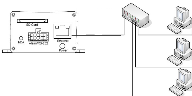
Рисунок 1-4 Сетевое Подключение с Помощью Патч-Кабеля
