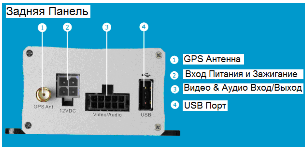
Рисунок 1-2 Задняя Панель
